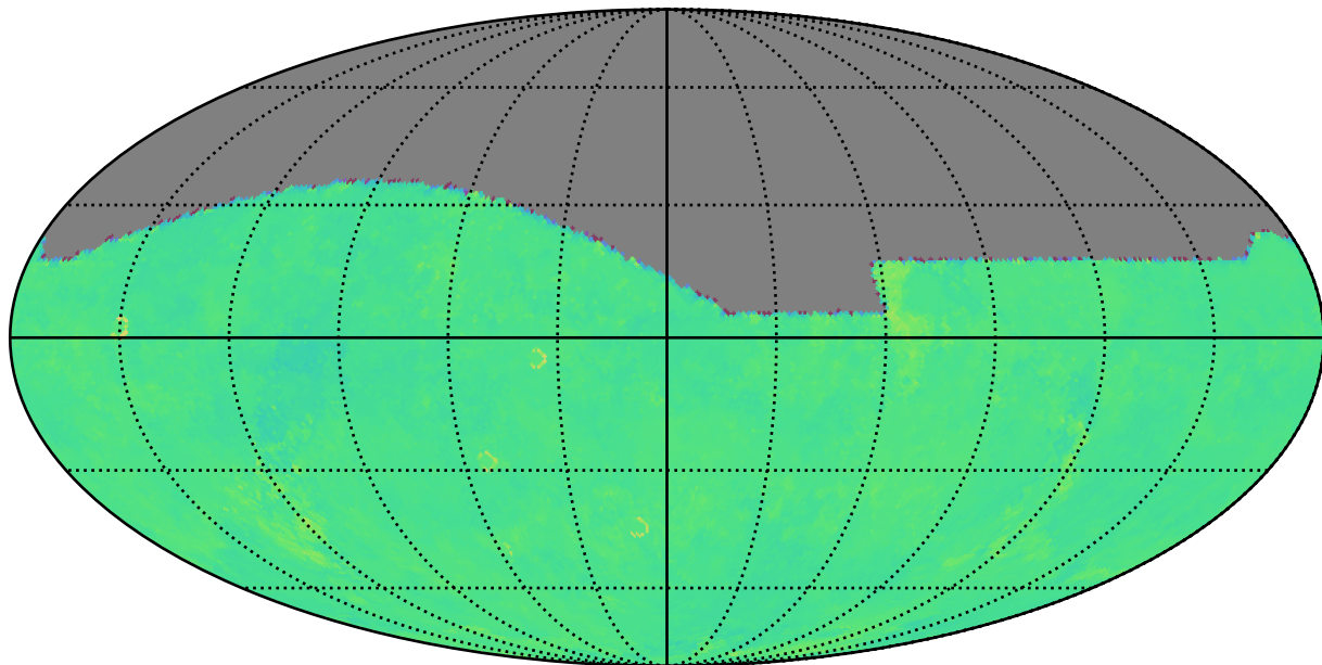
extra_ss_neo7_v3.4_10yrs g: Kuiper rotTelPos
