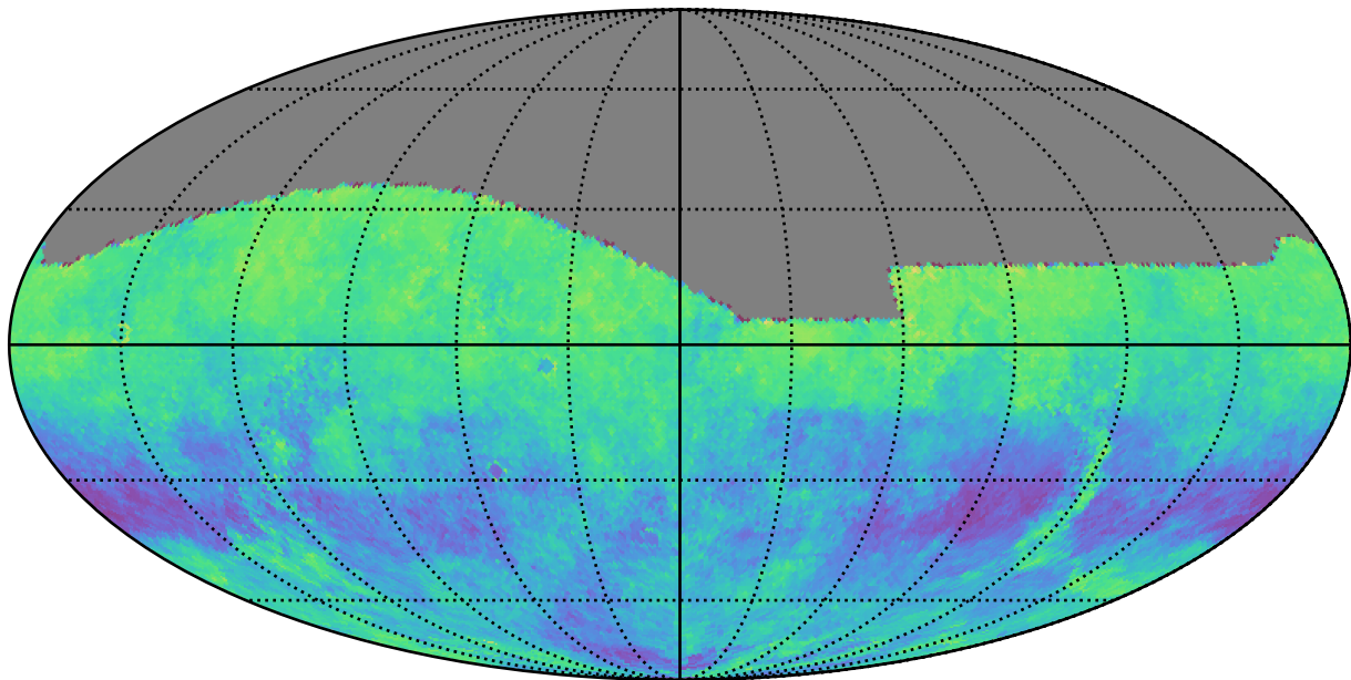
extra_ss_neo7_v3.4_10yrs g: Kuiper rotSkyPos
