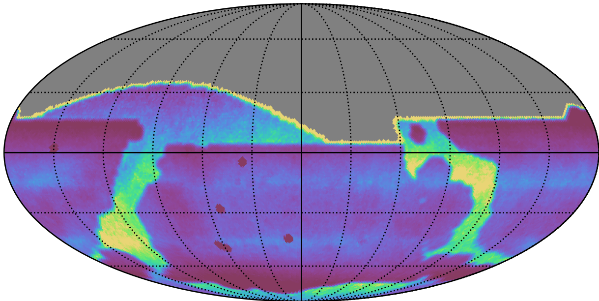
extra_ss_neo7_v3.4_10yrs : DCRprecision
