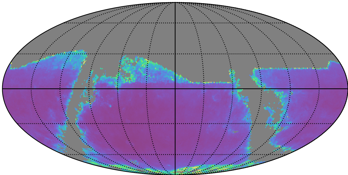
extra_ss_neo7_v3.4_10yrs r band: AGN SF_uncert
