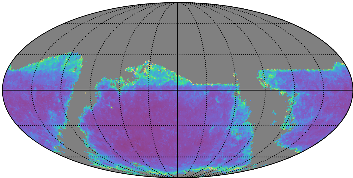
extra_ss_neo7_v3.4_10yrs g band: AGN SF_uncert
