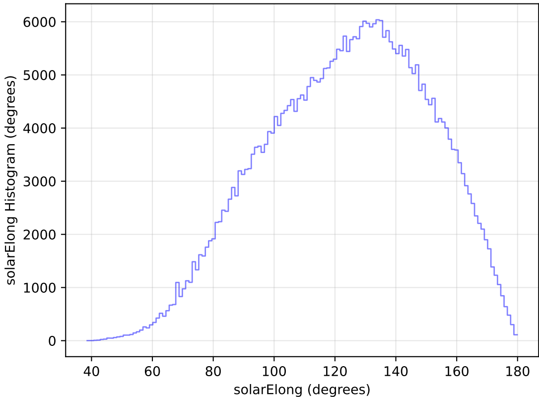
extra_ss_neo7_v3.4_10yrs WFD y band: solarElong Histogram
