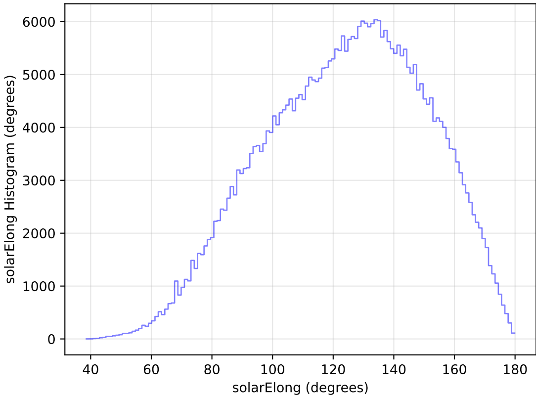
extra_ss_neo7_v3.4_10yrs All sky y band: solarElong Histogram
