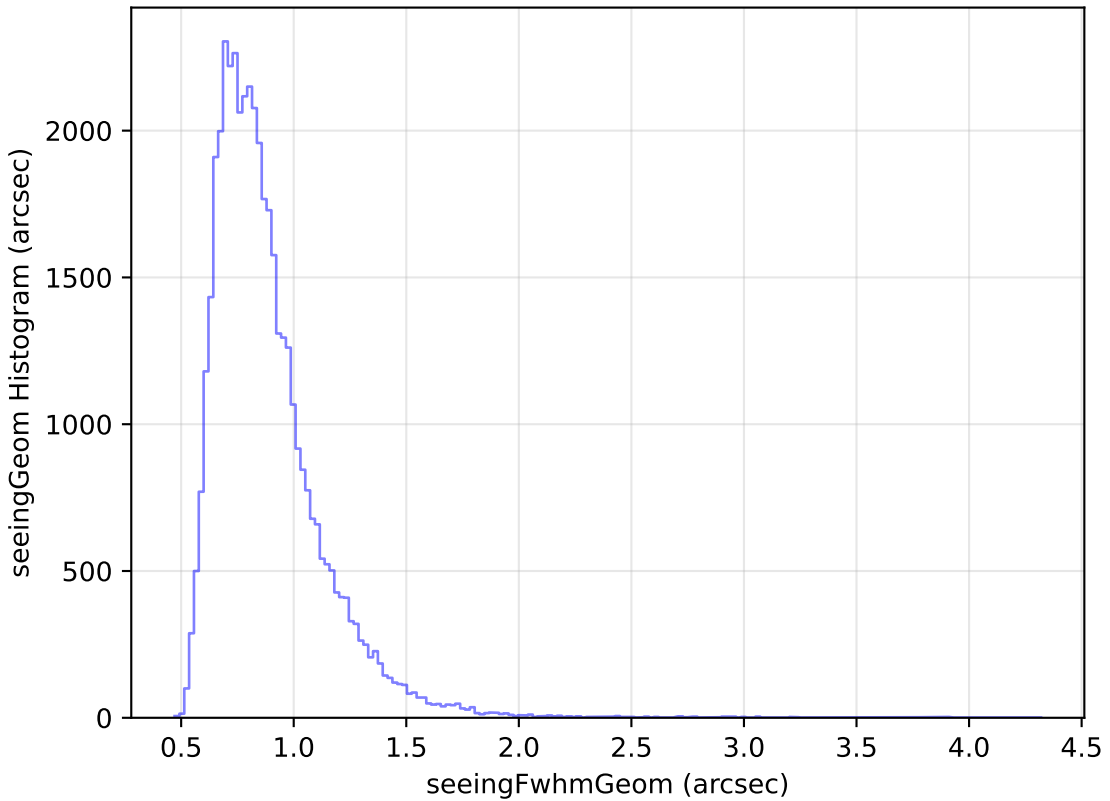
extra_ss_neo7_v3.4_10yrs Yr 1 z band: seeingGeom Histogram
