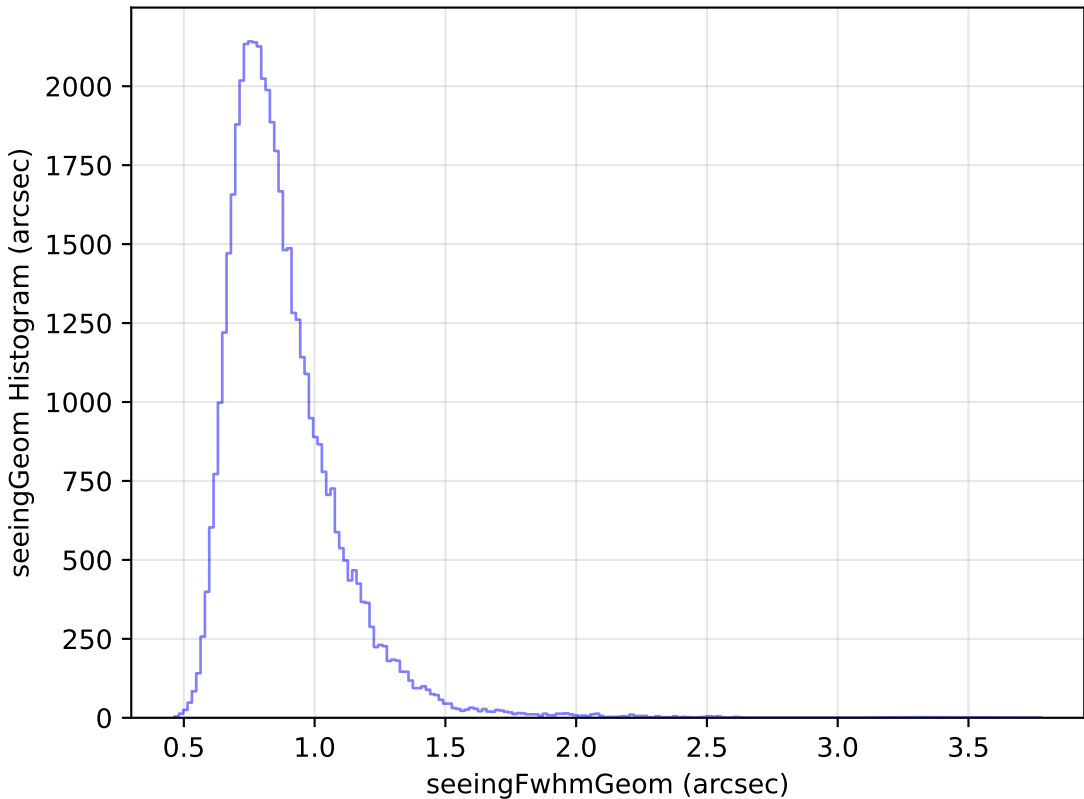
extra_ss_neo7_v3.4_10yrs Yr 1 y band: seeingGeom Histogram
