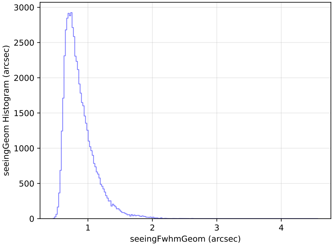
extra_ss_neo7_v3.4_10yrs Yr 1 i band: seeingGeom Histogram
