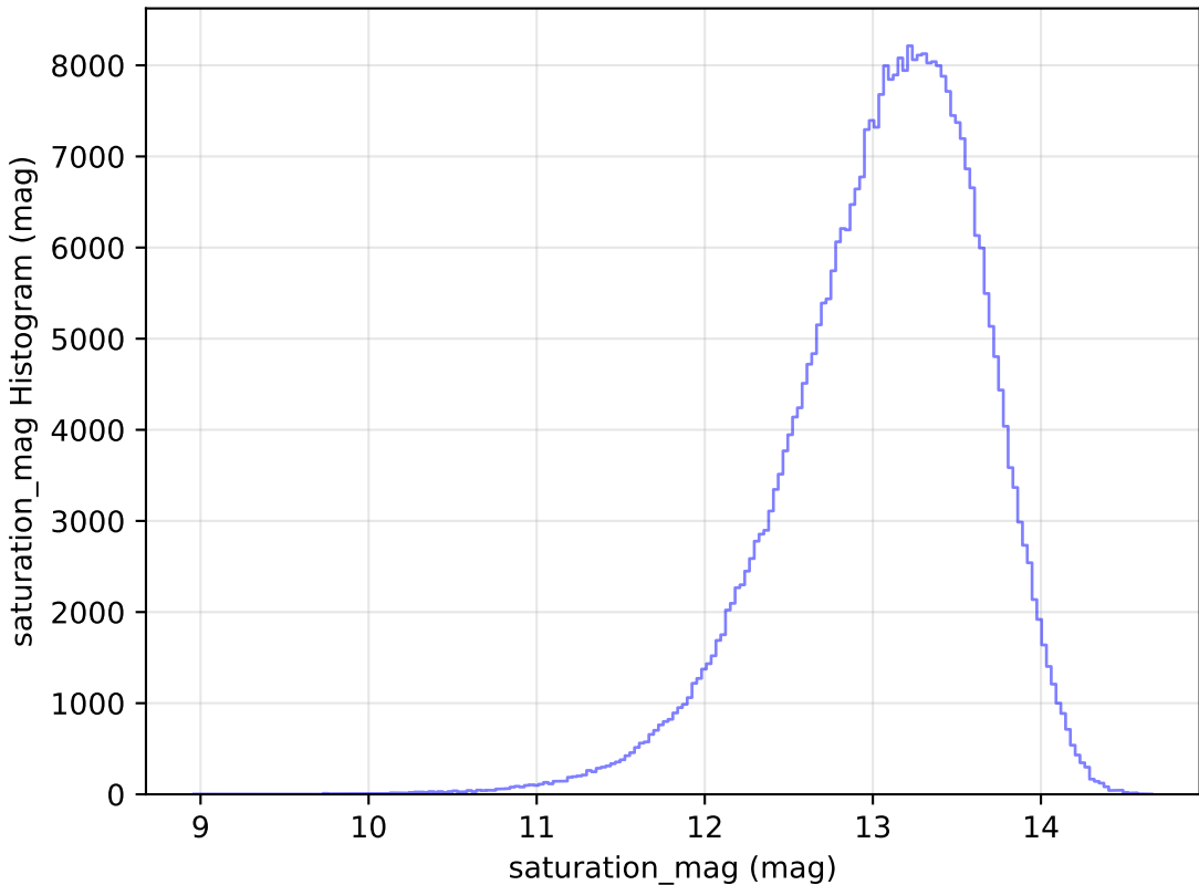
extra_ss_neo7_v3.4_10yrs All sky y band: saturation_mag Histogram
