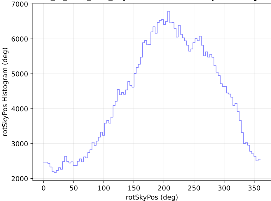
extra_ss_neo7_v3.4_10yrs WFD z band: rotSkyPos Histogram
