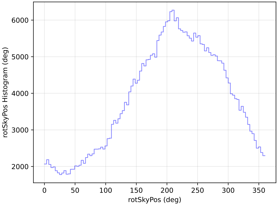
extra_ss_neo7_v3.4_10yrs WFD y band: rotSkyPos Histogram
