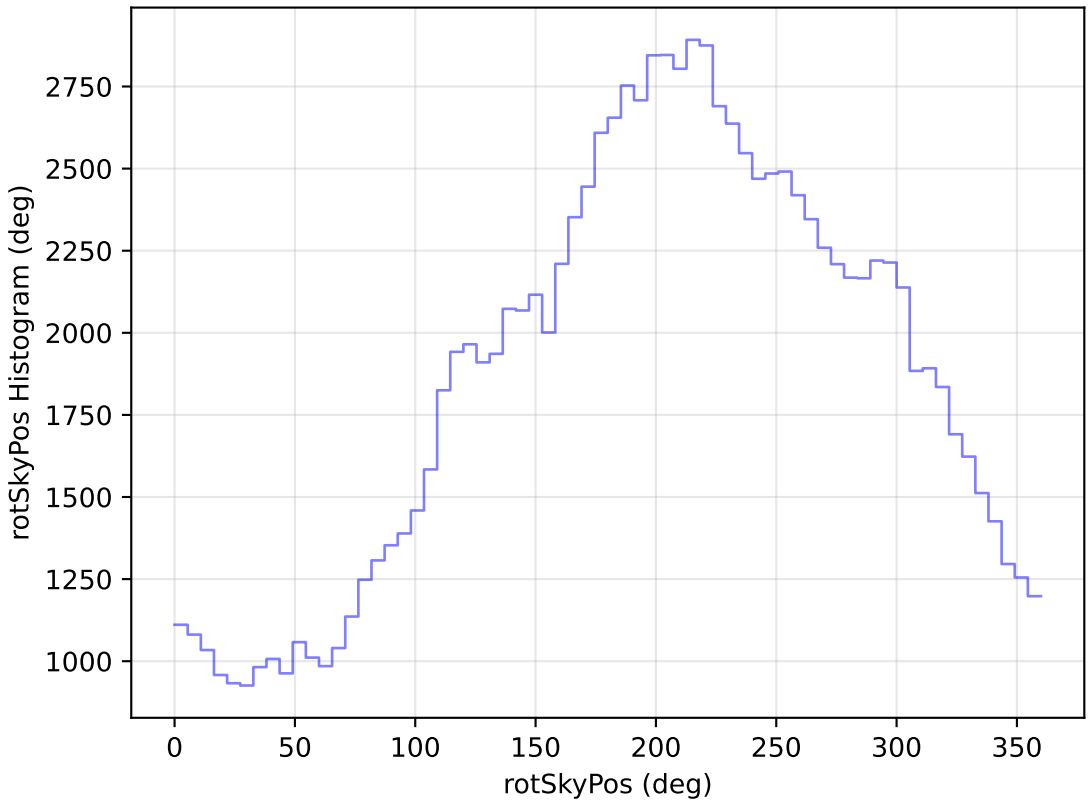
extra_ss_neo7_v3.4_10yrs WFD u band: rotSkyPos Histogram
