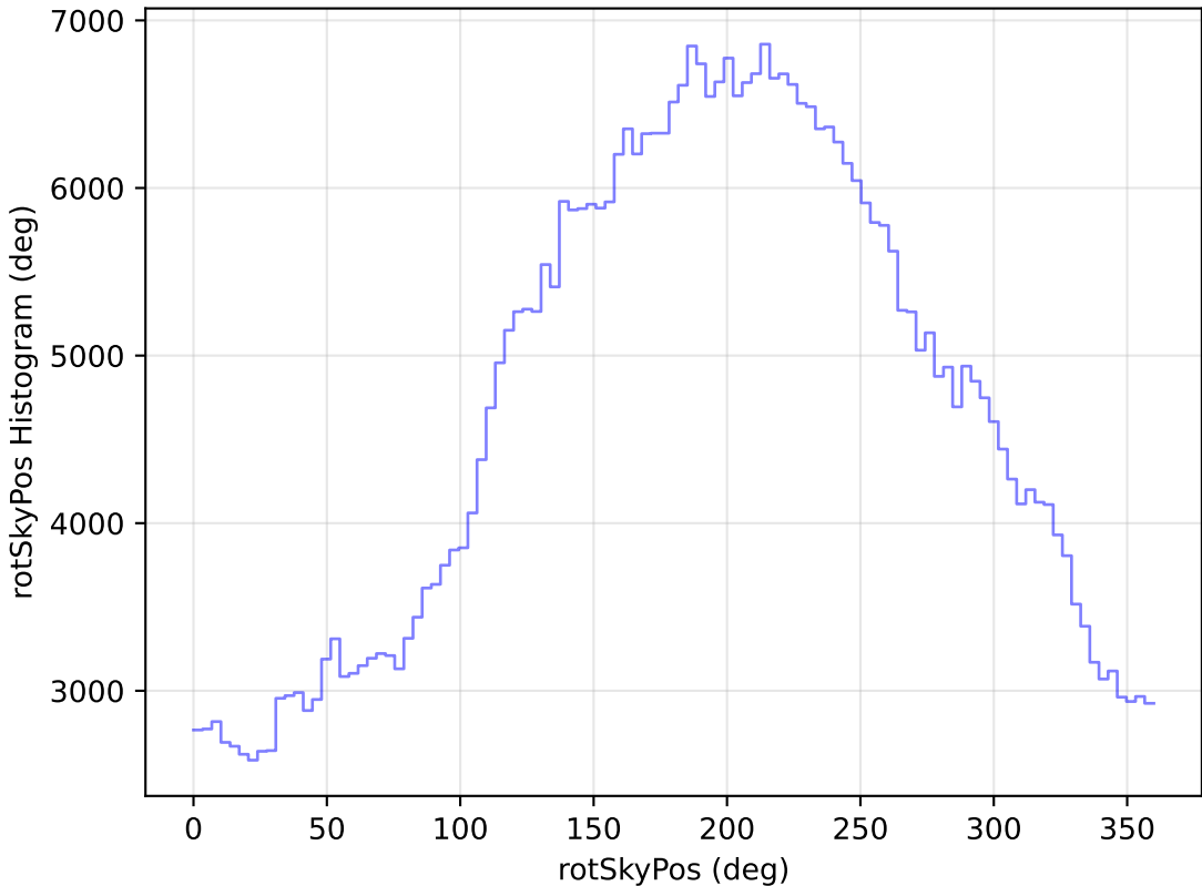
extra_ss_neo7_v3.4_10yrs WFD r band: rotSkyPos Histogram
