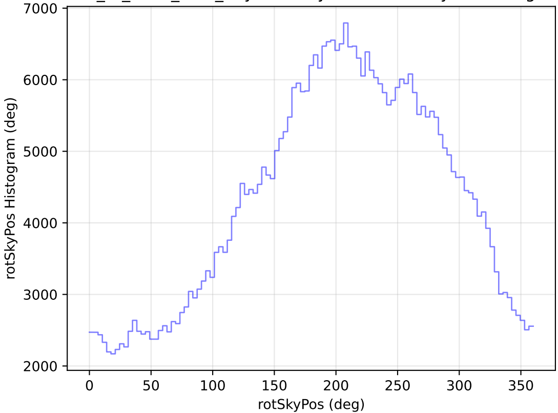
extra_ss_neo7_v3.4_10yrs All sky z band: rotSkyPos Histogram
