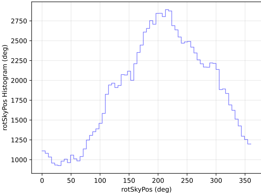
extra_ss_neo7_v3.4_10yrs All sky u band: rotSkyPos Histogram
