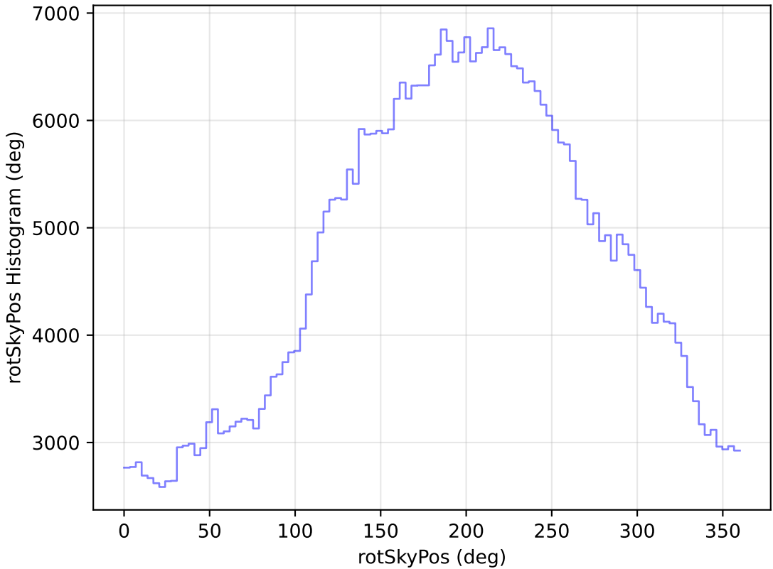
extra_ss_neo7_v3.4_10yrs All sky r band: rotSkyPos Histogram
