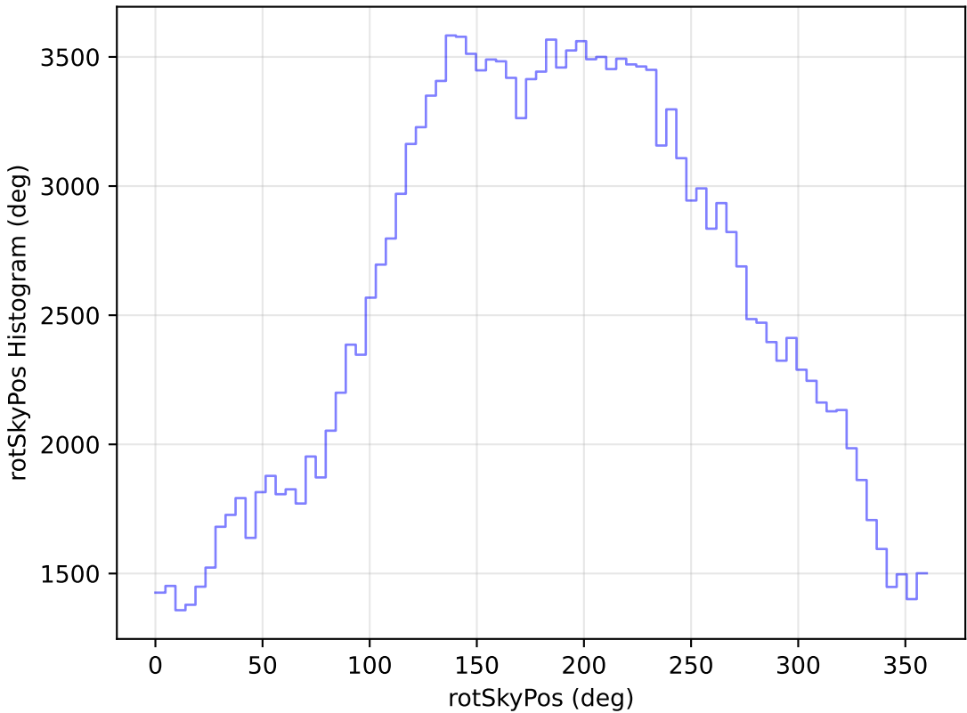
extra_ss_neo7_v3.4_10yrs All sky g band: rotSkyPos Histogram
