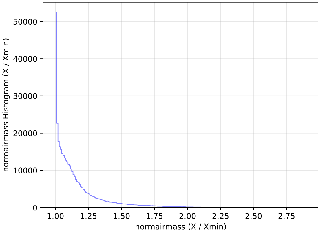
extra_ss_neo7_v3.4_10yrs WFD y band: normairmass Histogram
