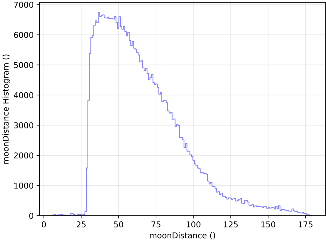
extra_ss_neo7_v3.4_10yrs All sky y band: moonDistance Histogram
