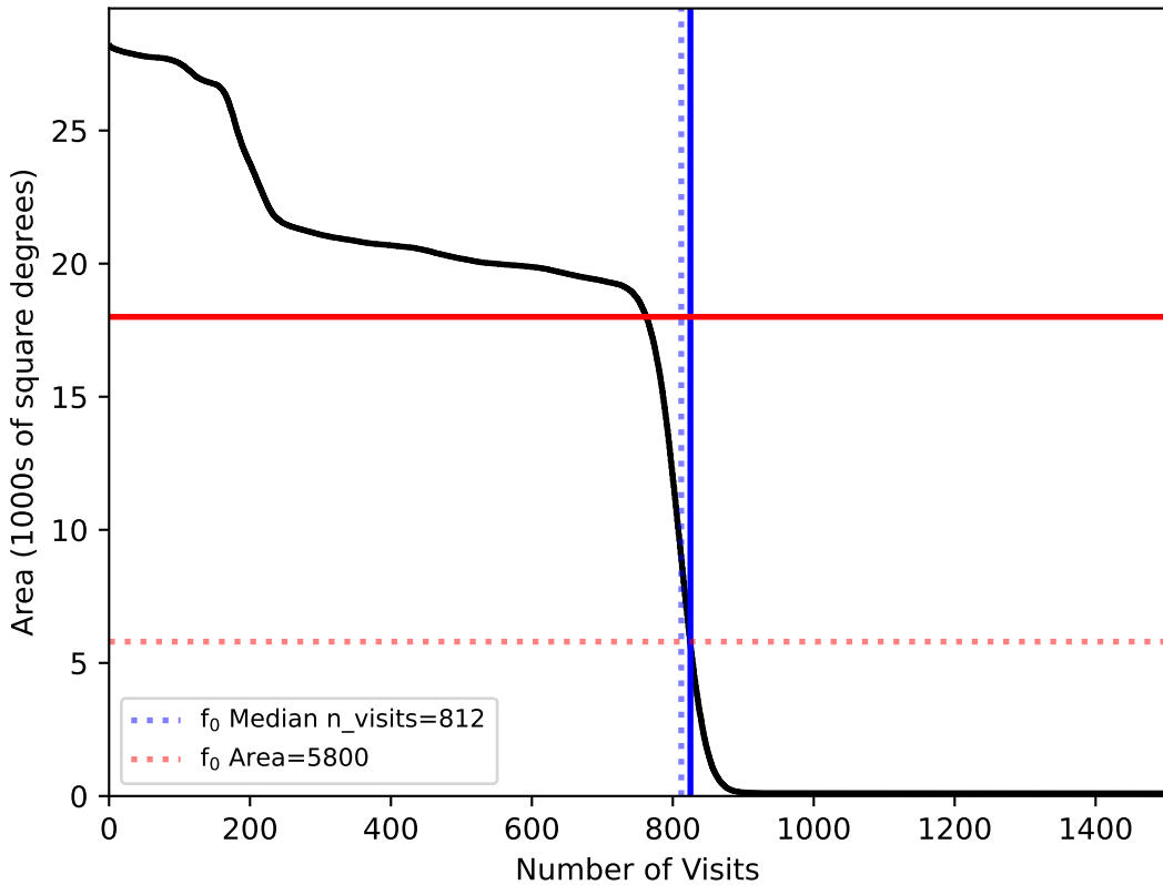
extra_ss_neo7_v3.4_10yrs All sky: fO
