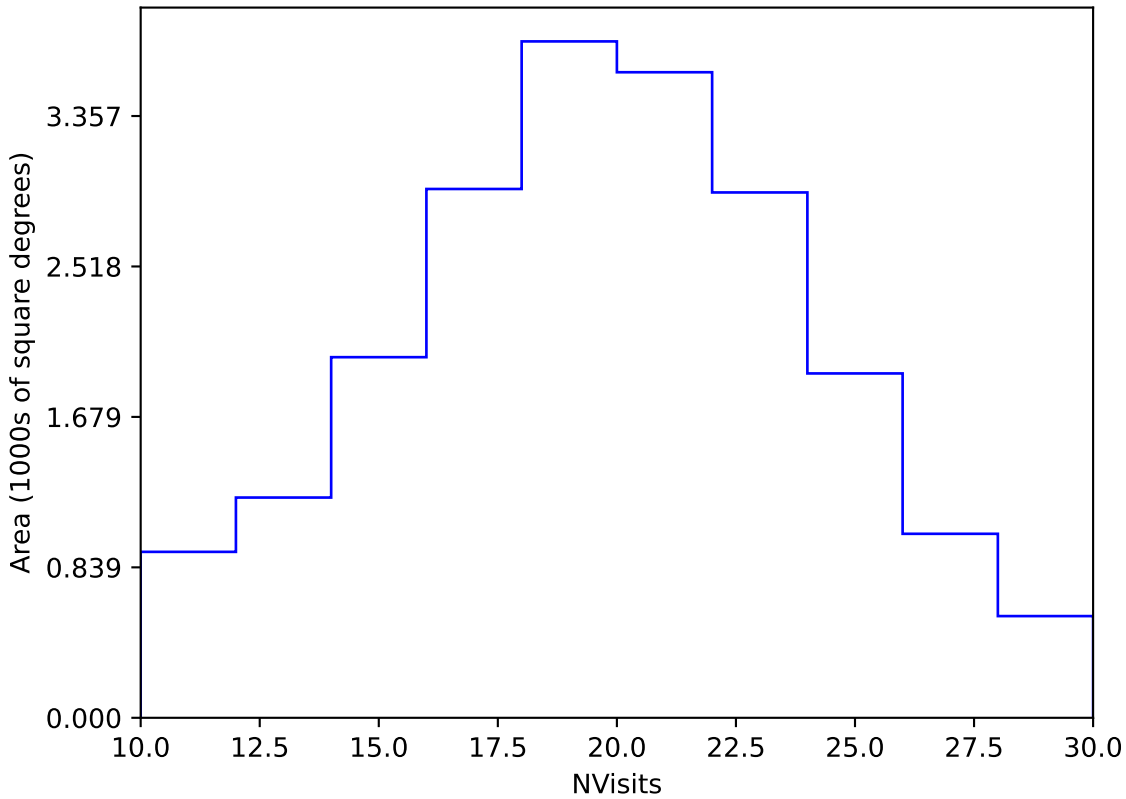
extra_ss_neo7_v3.4_10yrs Yr 1 y band: NVisits
