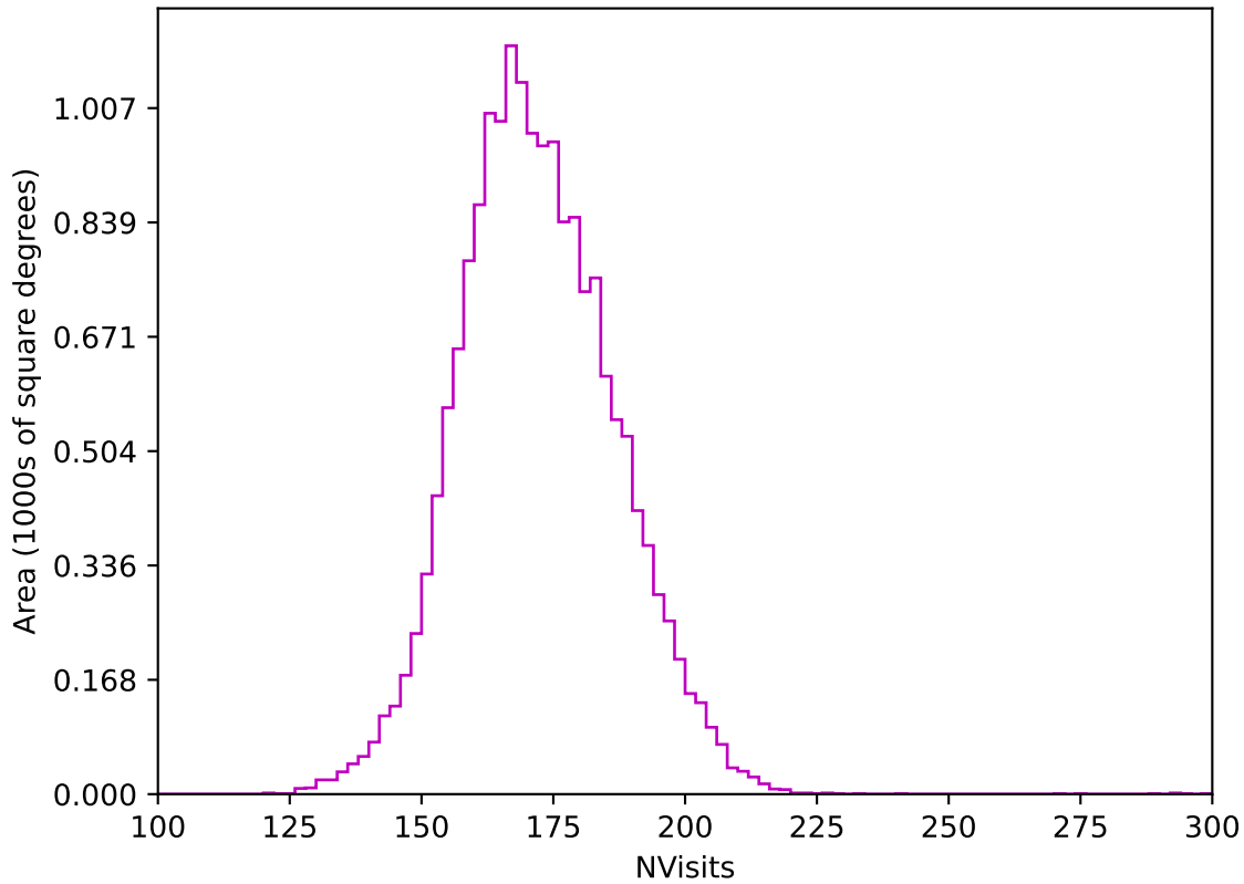
extra_ss_neo7_v3.4_10yrs WFD z band: NVisits
