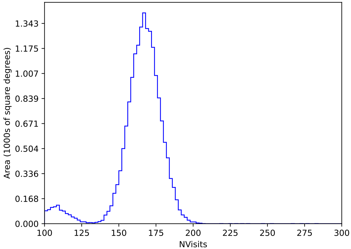
extra_ss_neo7_v3.4_10yrs WFD y band: NVisits
