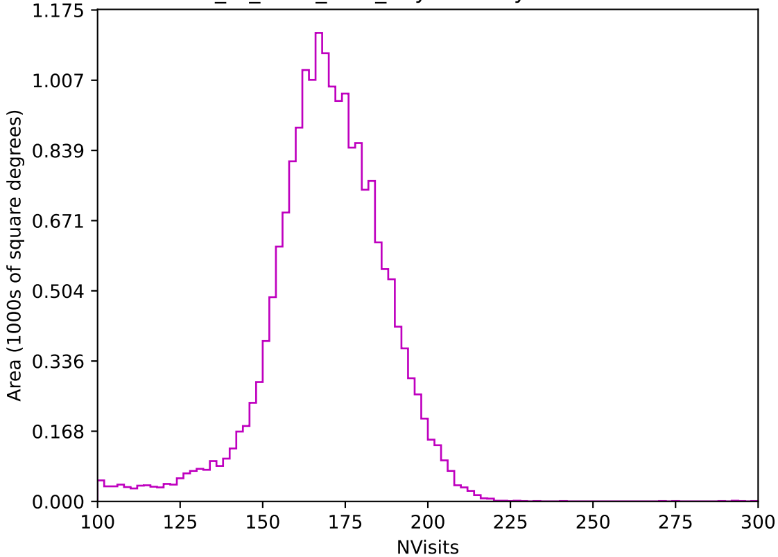
extra_ss_neo7_v3.4_10yrs All sky z band: NVisits
