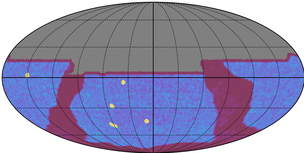
extra_ss_neo7_v3.4_10yrs All sky y band: NVisits
