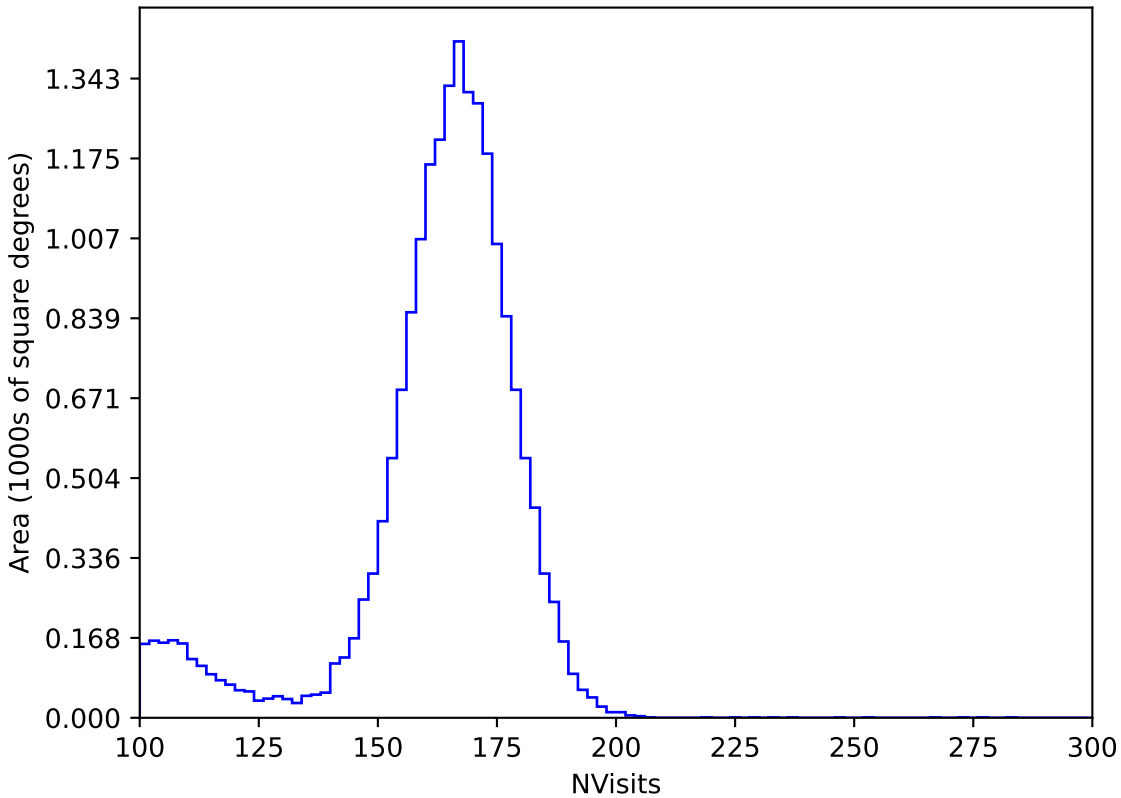
extra_ss_neo7_v3.4_10yrs All sky y band: NVisits
