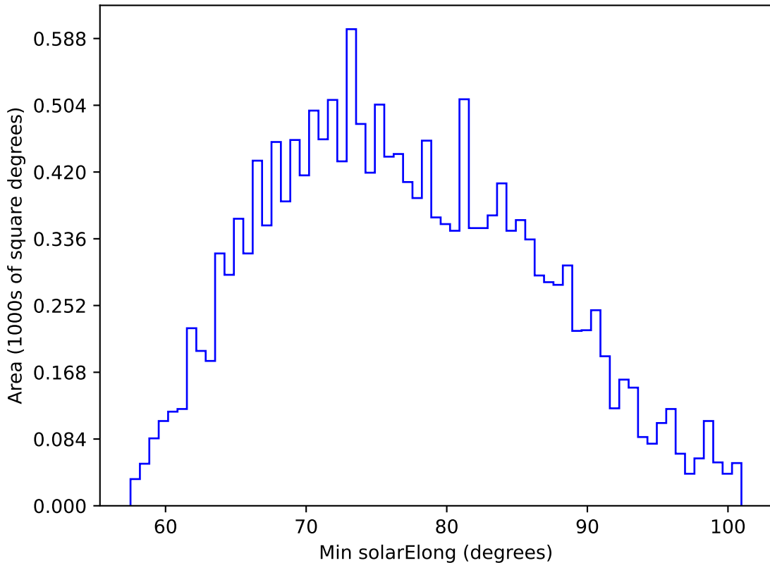
extra_ss_neo7_v3.4_10yrs WFD u band: Min solarElong
