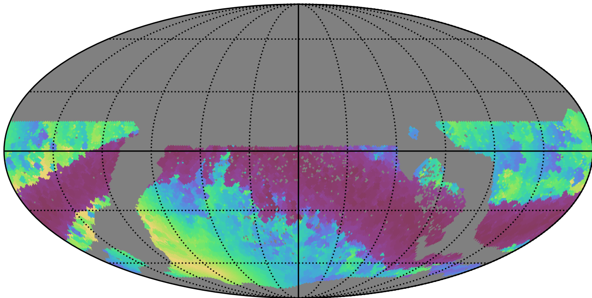
extra_ss_neo7_v3.4_10yrs WFD r band: Min solarElong
