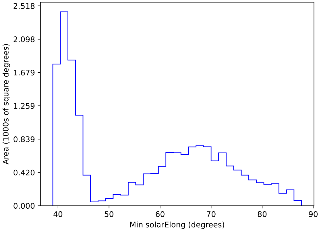
extra_ss_neo7_v3.4_10yrs WFD r band: Min solarElong
