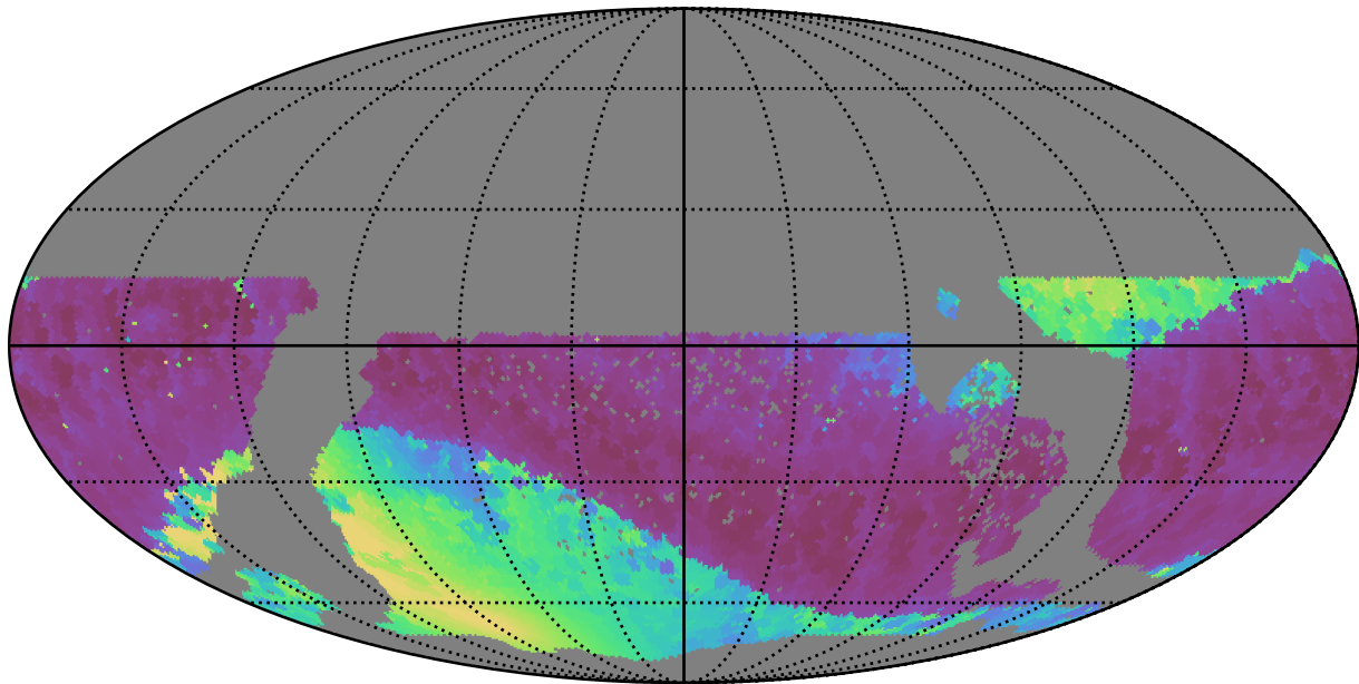
extra_ss_neo7_v3.4_10yrs WFD i band: Min solarElong
