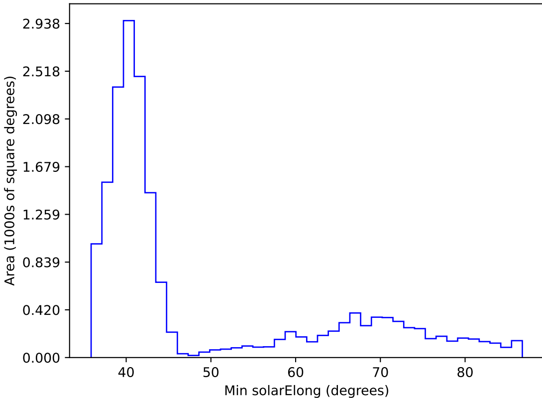
extra_ss_neo7_v3.4_10yrs WFD i band: Min solarElong
