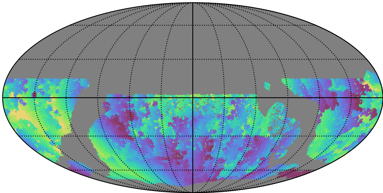
extra_ss_neo7_v3.4_10yrs WFD g band: Min solarElong
