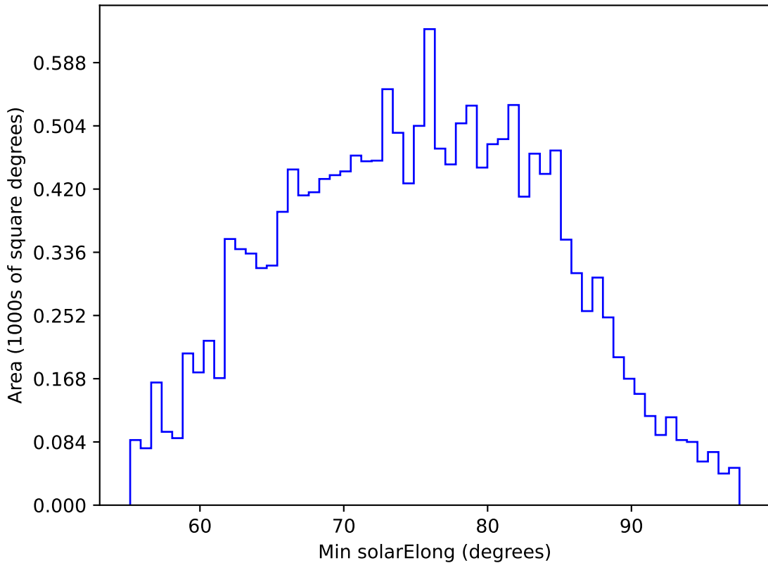
extra_ss_neo7_v3.4_10yrs WFD g band: Min solarElong
