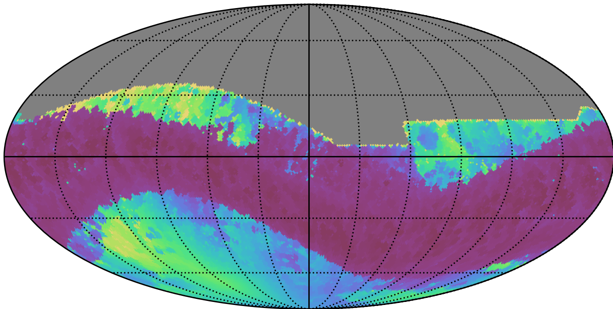
extra_ss_neo7_v3.4_10yrs All sky z band: Min solarElong
