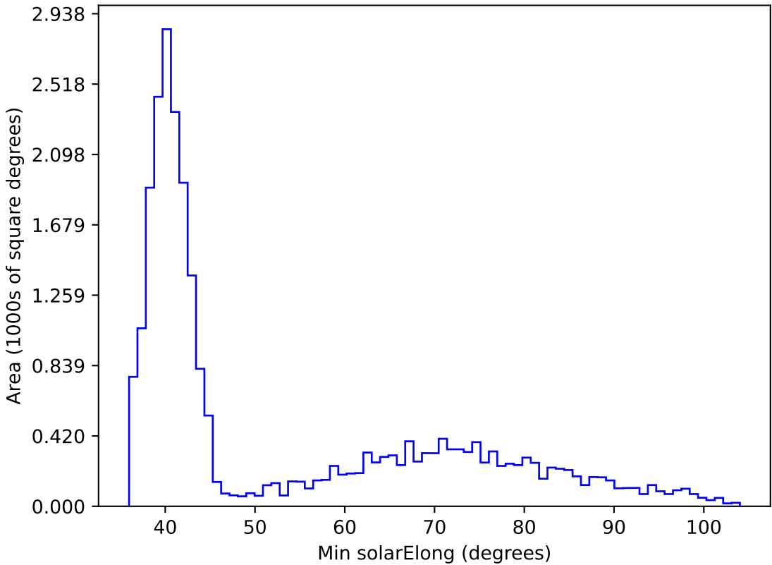
extra_ss_neo7_v3.4_10yrs All sky z band: Min solarElong
