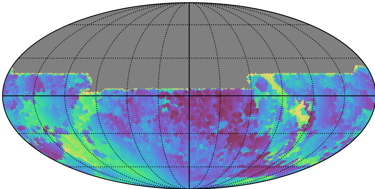
extra_ss_neo7_v3.4_10yrs All sky y band: Min solarElong
