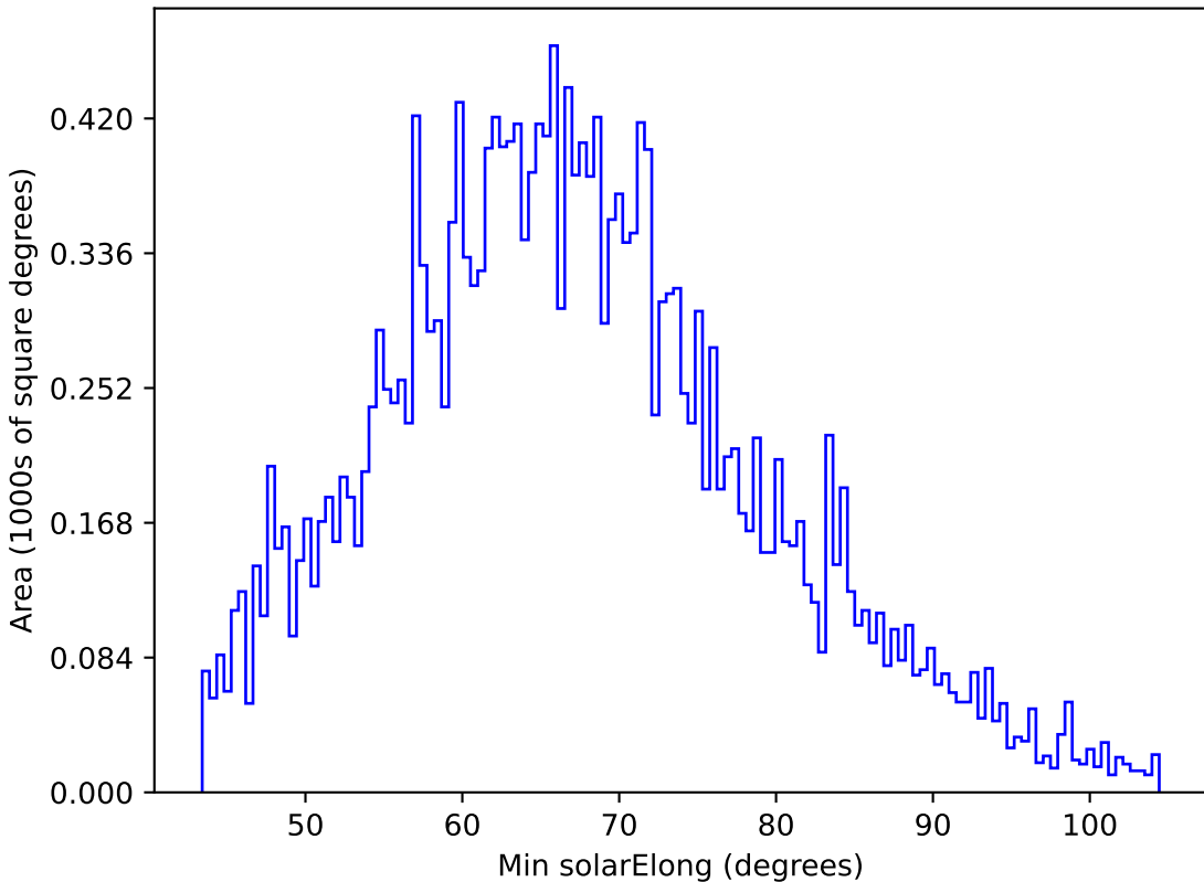
extra_ss_neo7_v3.4_10yrs All sky y band: Min solarElong
