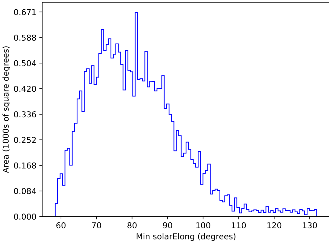
extra_ss_neo7_v3.4_10yrs All sky u band: Min solarElong
