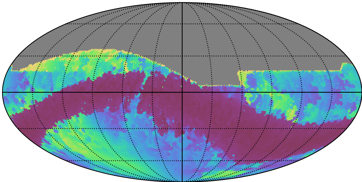
extra_ss_neo7_v3.4_10yrs All sky r band: Min solarElong
