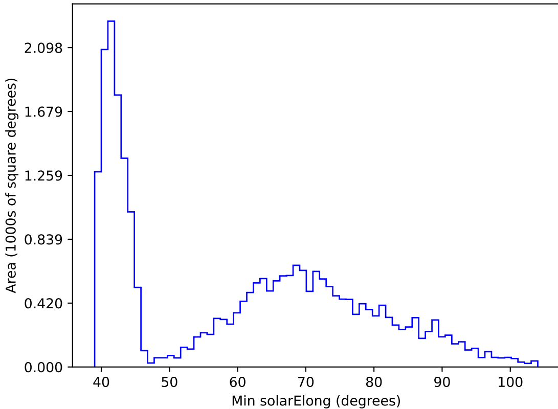
extra_ss_neo7_v3.4_10yrs All sky r band: Min solarElong
