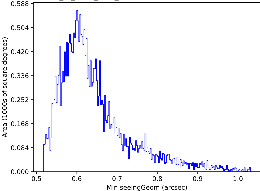
extra_ss_neo7_v3.4_10yrs Yr 1 z band: Min seeingGeom
