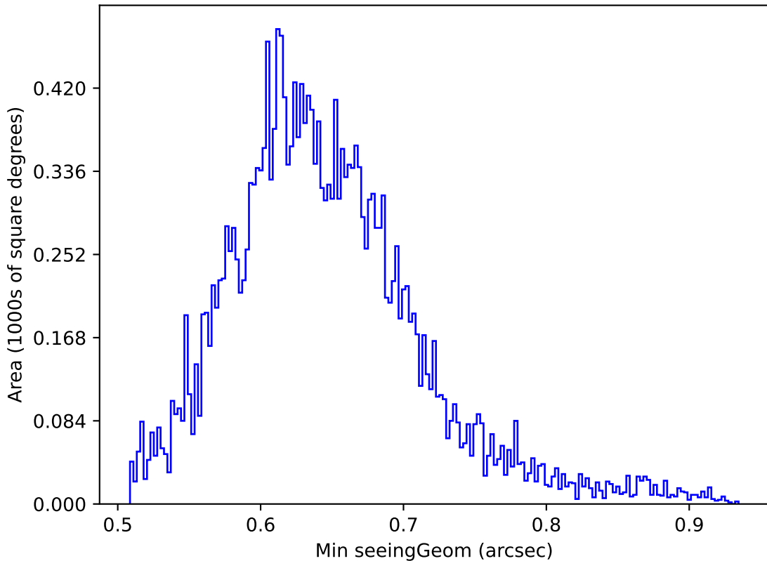
extra_ss_neo7_v3.4_10yrs Yr 1 y band: Min seeingGeom
