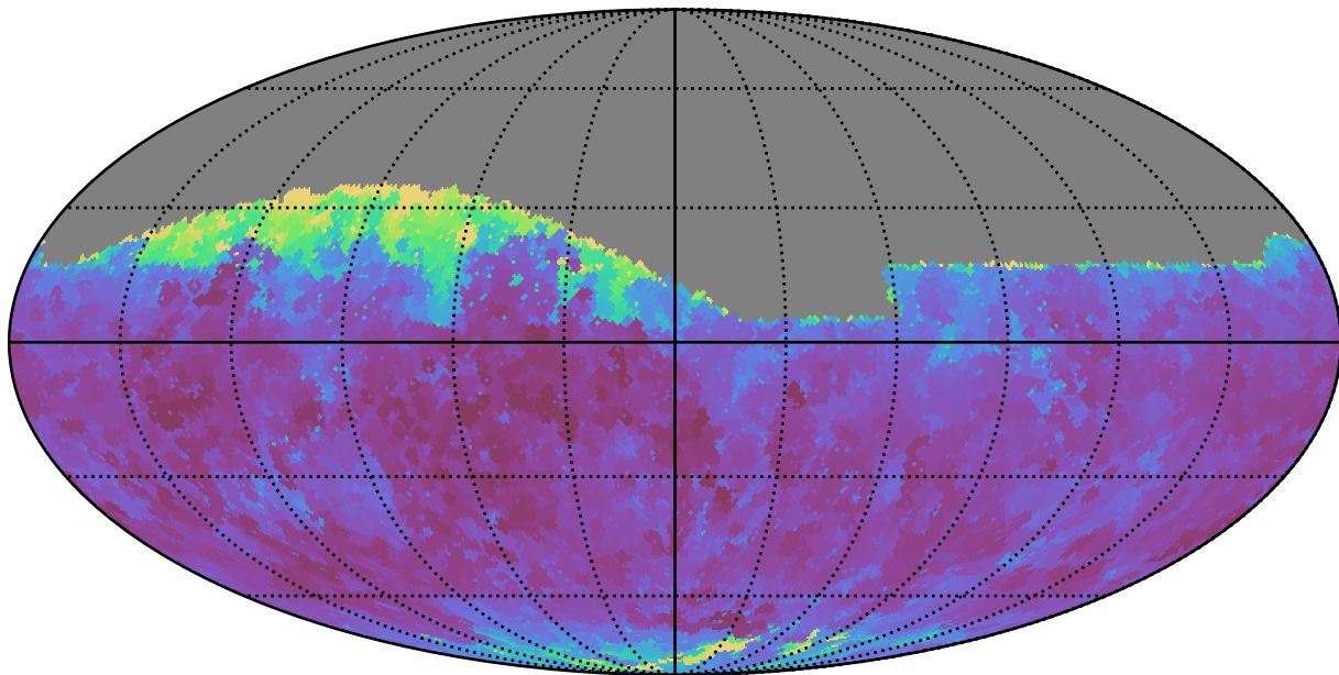
extra_ss_neo7_v3.4_10yrs Yr 1 r band: Min seeingGeom
