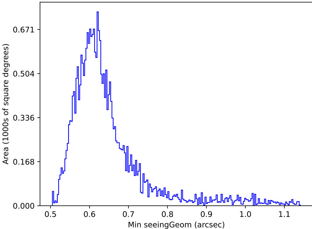
extra_ss_neo7_v3.4_10yrs Yr 1 r band: Min seeingGeom
