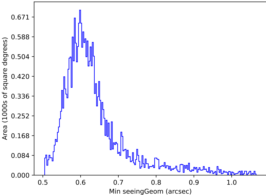
extra_ss_neo7_v3.4_10yrs Yr 1 i band: Min seeingGeom
