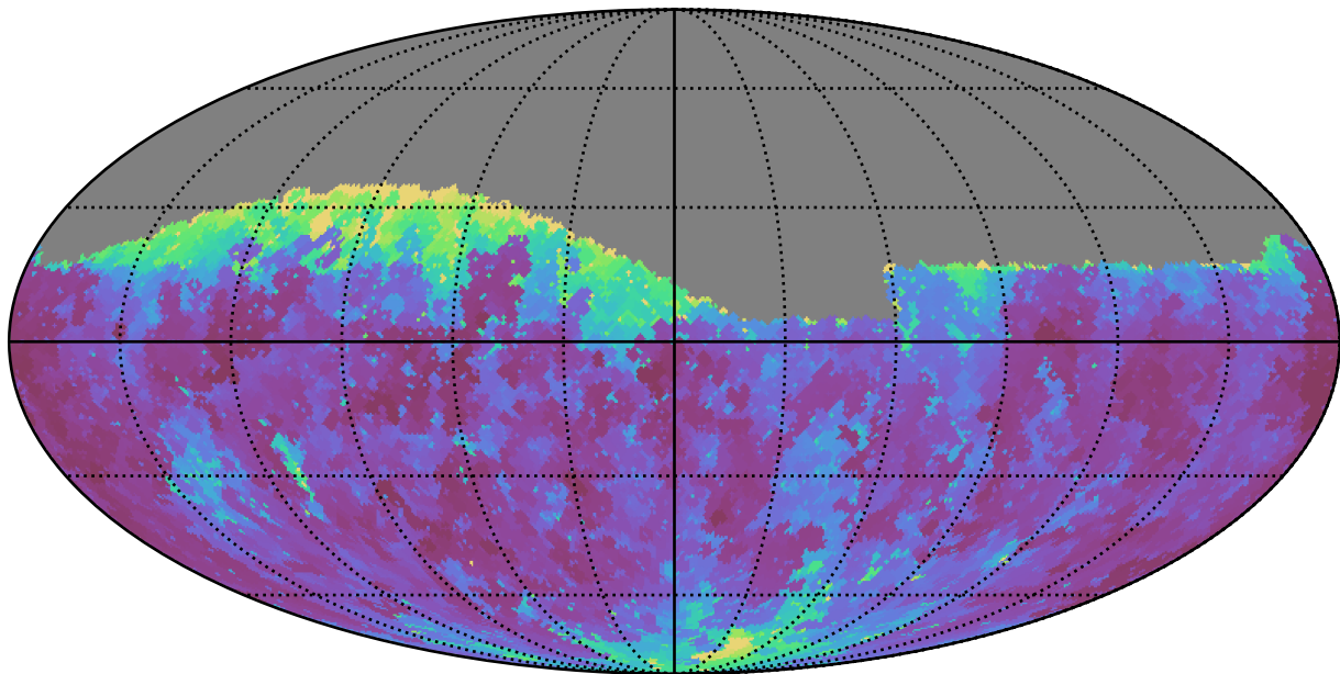
extra_ss_neo7_v3.4_10yrs Yr 1 g band: Min seeingGeom
