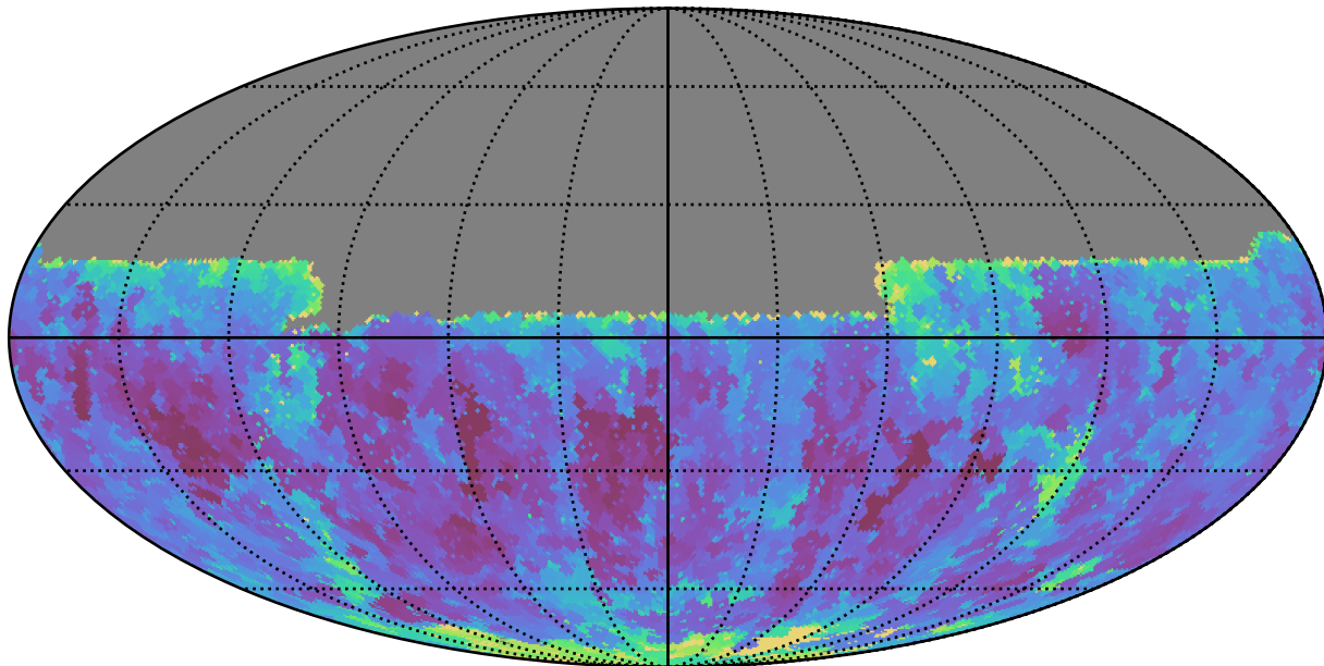
extra_ss_neo7_v3.4_10yrs Yr 1 y band: Min seeingEff
