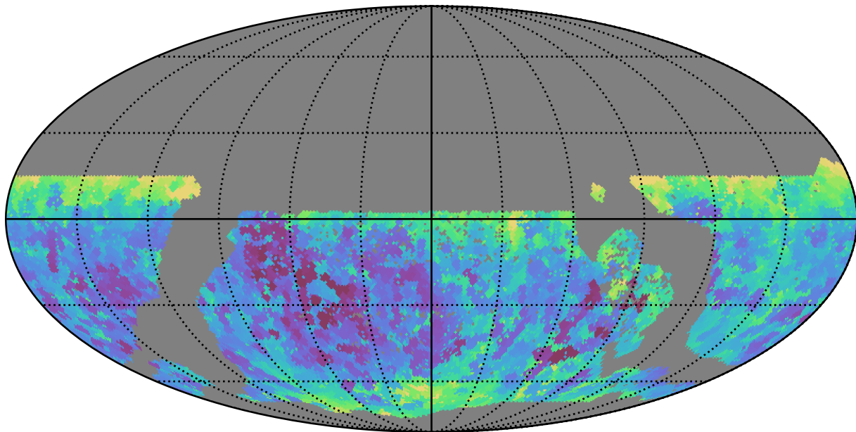
extra_ss_neo7_v3.4_10yrs WFD y band: Min seeingEff
